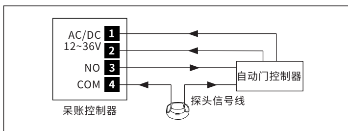
呆账控制器控制感应器接线图
