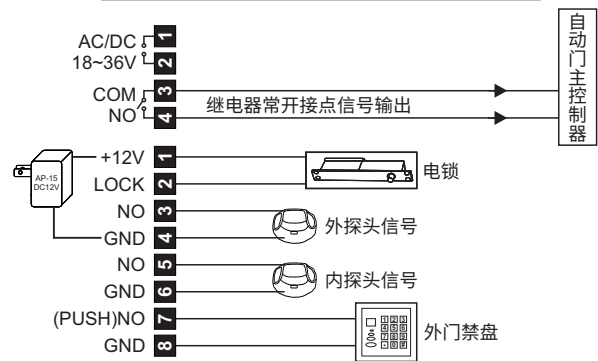
外接DC12V稳压电源接法示意图
